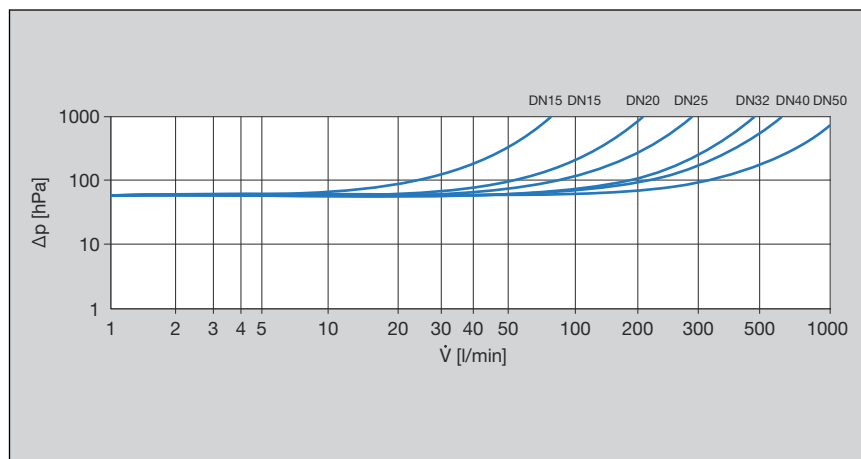
Bild 1: Prestandadiagram tryckförlust backskydd press-/gänganslutning
