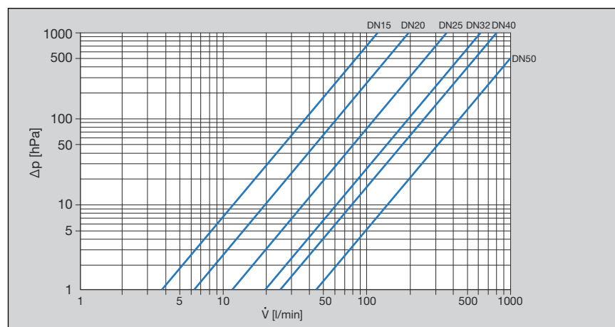
Bild 1: Prestandadiagram snedsättesventiler press-/gånganslutning
