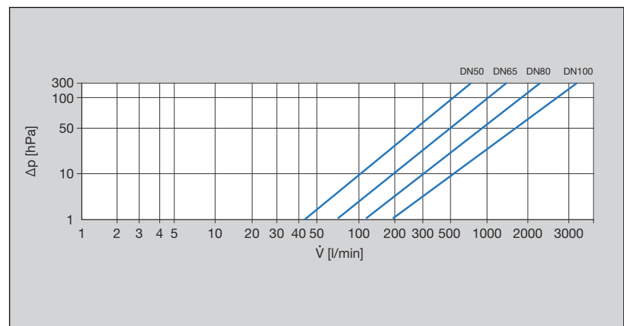
Bild 1: Prestandadiagram tryckförlust KRV XL-snedsätesventiler flänsanslutning
