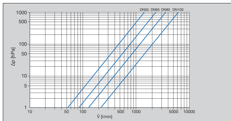
Bild 1: Prestandadiagram tryckförlust XL-snedsättesventiler flänsanslutning
