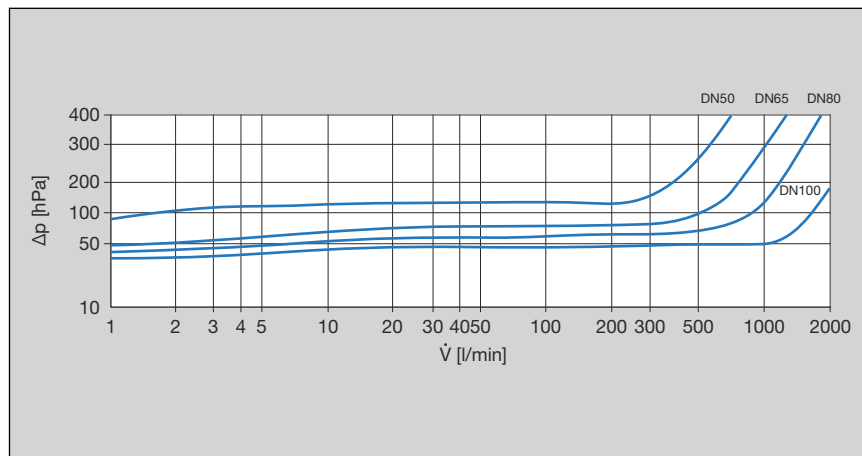
Bild 1: Prestandadiagram tryckförlust backskydd flänsanslutning
