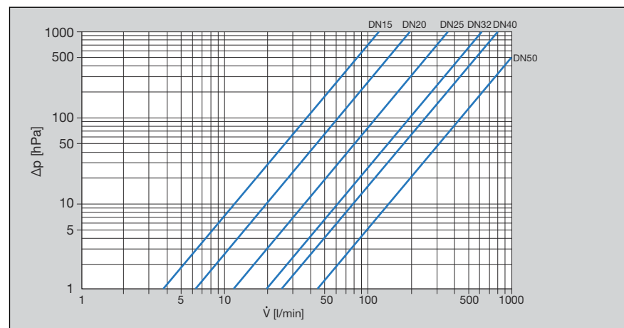
Bild 3: Prestandadiagram snedsättesventiler press-/gånganslutning
