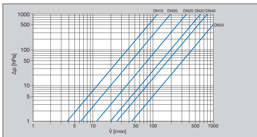
Bild 1: Prestandadiagram snedsättesventiler press-/gånganslutning
