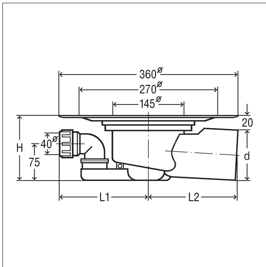
Bild 6: Ritning för modell 4955.15
