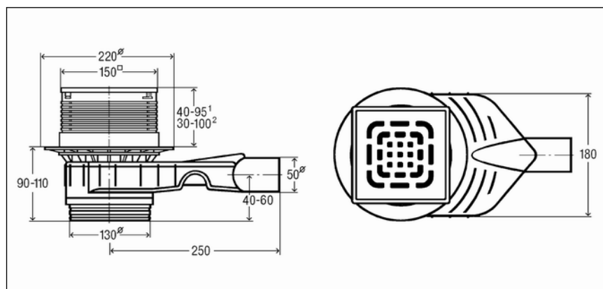
Bild 8: Ritning modell 4914.11
