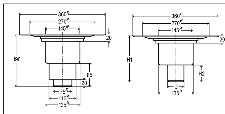
Bild 5: Ritning modell 4951.15
