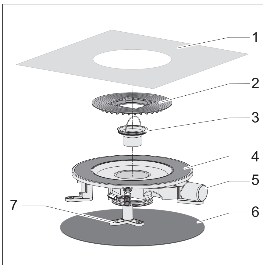
Bild 1: Leveransomfattning modell 4914.2
