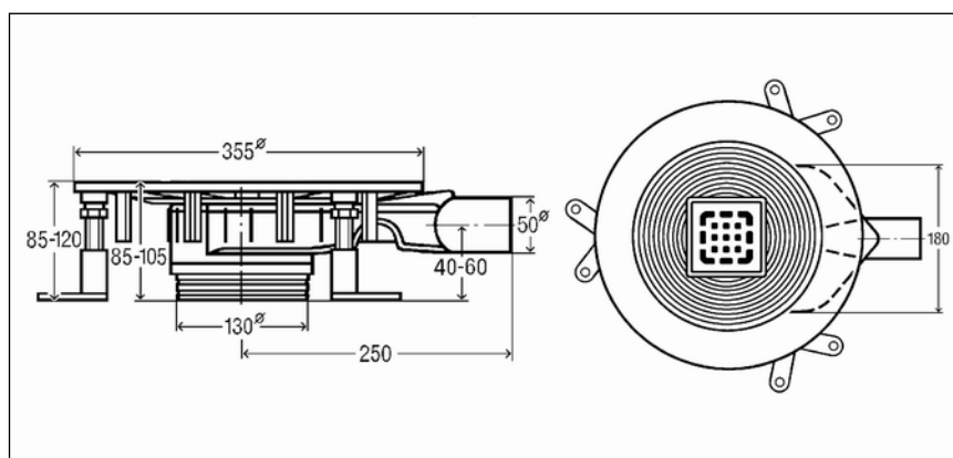
Bild 7: Ritning modell 4914.2
