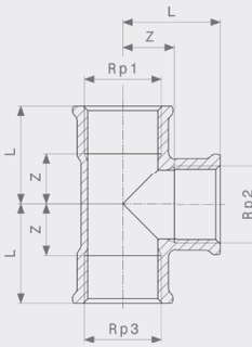
T-rör - mässing Modell 1622
