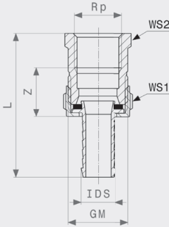
Skruvförband för stigarrör - mässing Modell 1841
