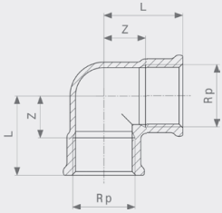
Böj 90° - mässing Modell 1612
