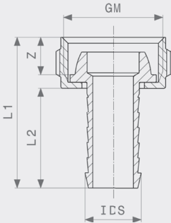
Slangkruvförband - mässing Modell 1812
