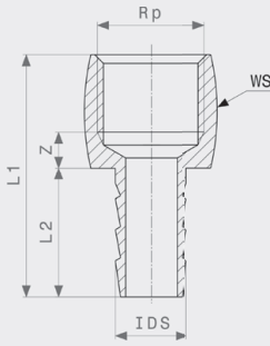
Slangmunstycke - mässing Modell 1846
