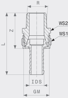
Skruvförband för stigarrör - mässing Modell 1832
