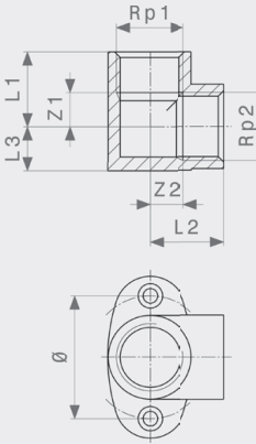
Ventilfäste - mässing Modell 1421
