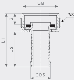
Slangkruvförband - mässing Modell 1811
