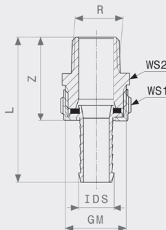
Skruvförband för stigarrör - mässing Modell 1831
