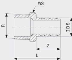
Slangmunstycke - mässing Modell 1845
