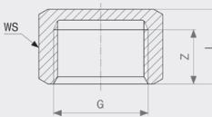
Huv - mässing Modell 1761
