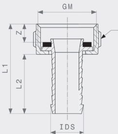
Slangkruvförband - mässing Modell 1814
