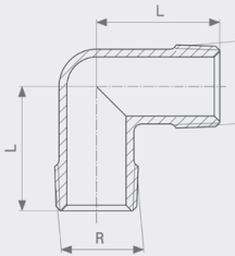
Böj 90° - mässing Modell 1611
