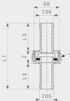
Slangkruvförband - mässing Modell 1821
