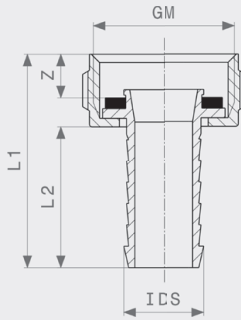
Slangkruvförband - mässing Modell 1817
