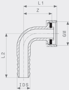
Slangkruvförband - mässing Modell 1813
