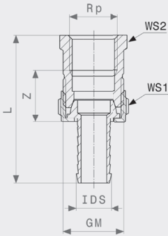
Skruvförband för stigarrör - mässing Modell 1842
