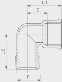
Böj 90° - mässing Modell 1613
