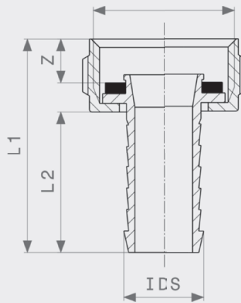
Slangkruvförband - mässing Modell 1819
