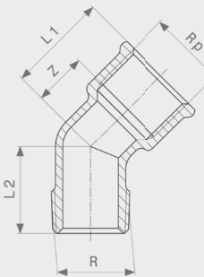
Böj 45° - mässing Modell 1615
