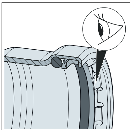
Slika 6: Narezni prsten
