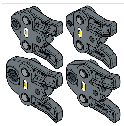
Obr. 5: lisovacie čeluste
