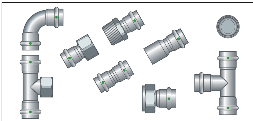
Obr. 1: lisované spojky Sanpress Inox
