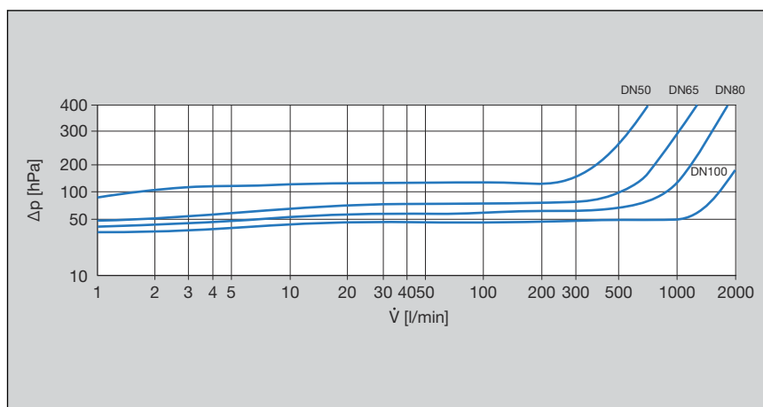
Obr. 1: Výkonový diagram - strata tlaku RV, prírubová prípojka
