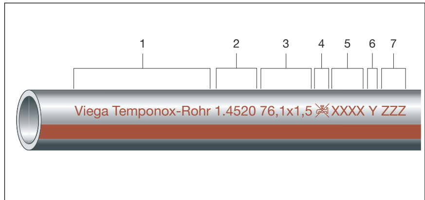
Fig. 6: Temponox pipe 1.4520
