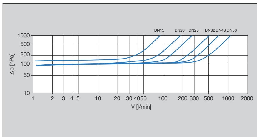
Fig. 3: Diagrama de desempenho Perda de pressão das KRV com conexão de prensar/rosca
