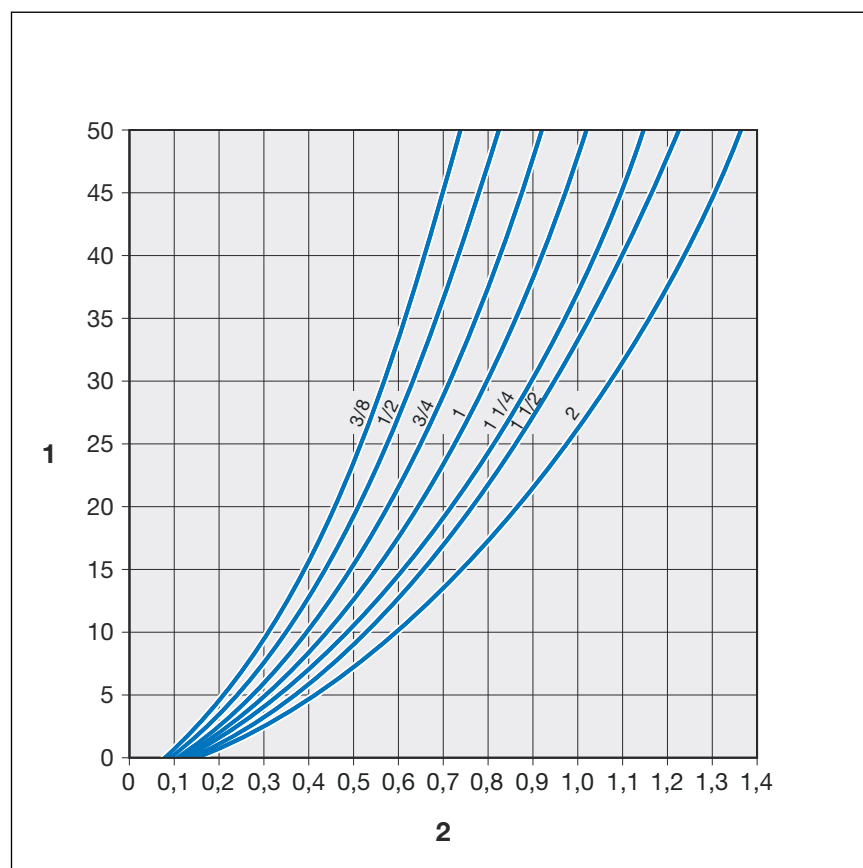
Fig. 7: Curvatura em forma de U para Megapress S \frac{3}{8} até 2 polegadas
