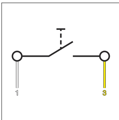
Fig. 2: Placa de acionamento para WC, ocupação da ligação para emissor de sinal externo
