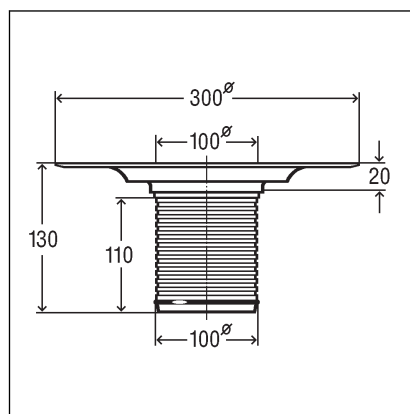
Rys. 4: Rysunek z wymiarami wzoru 4925
