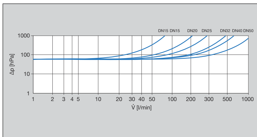
Rys. 3: Wykres charakterystyki: straty ciśnienia zaworu zwrotnego z przyłączem zaprasowywanym/gwintowym
