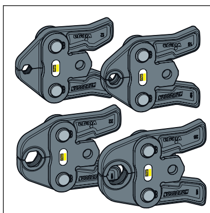
Rys. 11: Szczęki zaciskowe
