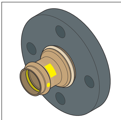
Rys. 6: Kołnierz ruchomy
