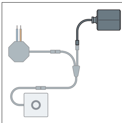
Schemat przyłączeniowy do redundantnego zasilania napięciem z pojemnikiem na baterie i zasilaczem.
