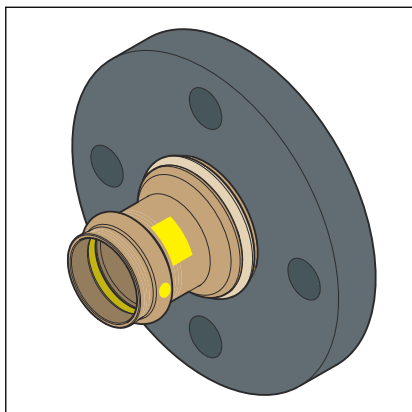
Fig. 6: Løs flens
