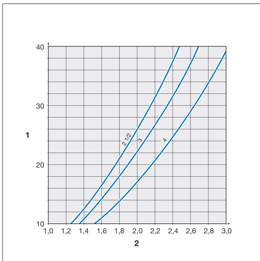
Fig. 5: Ekspansjonsbend Z- og T-form for Megapress S XL 2 1/2 til 4 tommer
