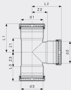
Seapress T-stykke - CuNiFe Modell 0318
