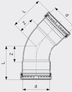
Seapress XL bend 45° - CuNiFe Modell 0326XL
