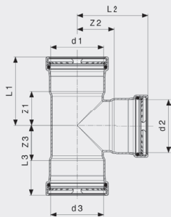
Seapress XL T-stykke - CuNiFe Modell 0318XL
