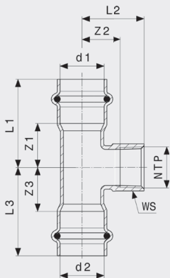
Seapress T-stykke - CuNiFe Modell 0317.5
