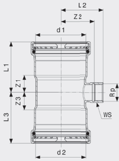
Seapress T-stykke - CuNiFe Modell 0317.2
