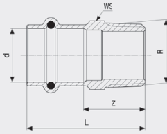
Profipress S nippelmuffe - rødgods eller silisiumbrønse Modell 4511
