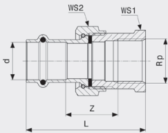
Profipress S union - rødgods eller silisiumbronse Modell 4562
