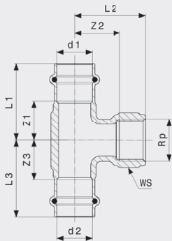
Profipress S T-stykke - rødgods eller silisiumbrøse Modell 4517.2
