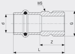
Profipress S nippelmuffe - rødgods eller silisiumbrønse Modell 4511.4
