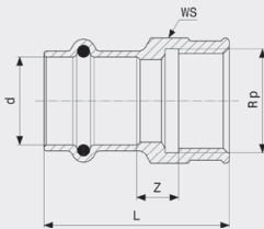
Profipress S overgangsmuffe - rødgods eller silisiumbrønse Modell 4512
