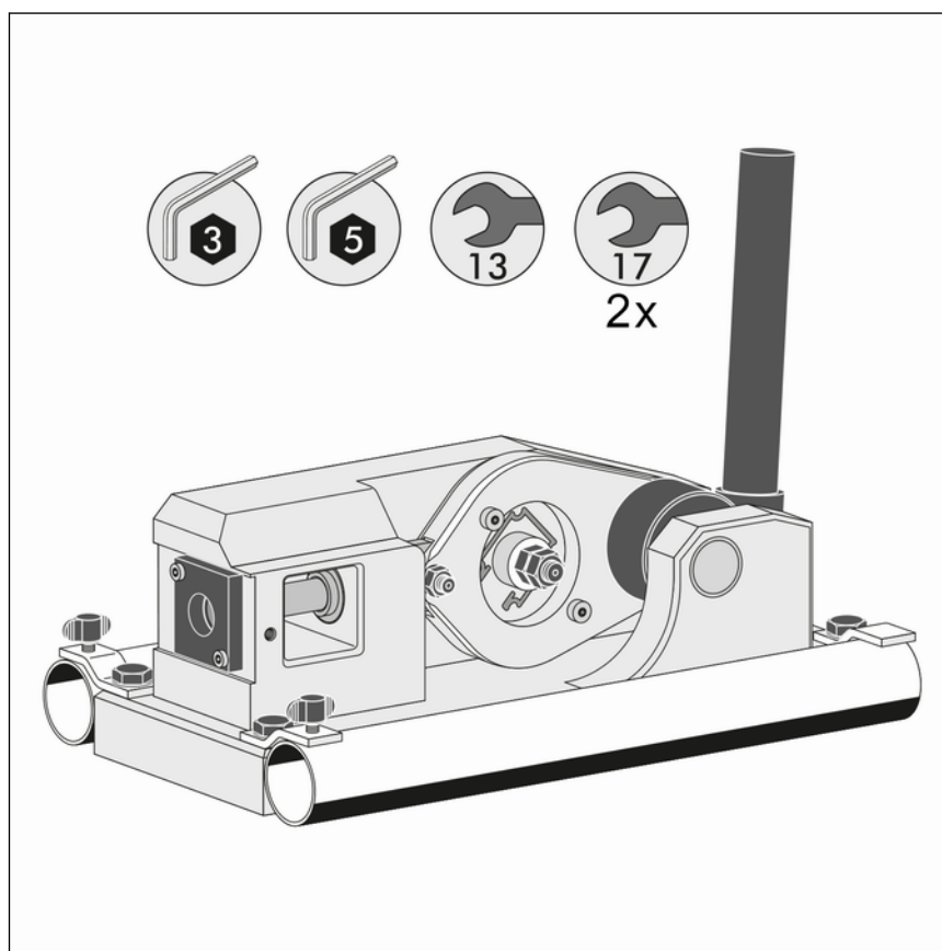
Afb. 2: Benodigd gereedschap
