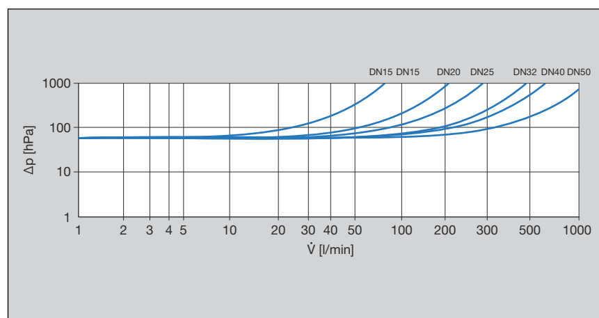
Afb. 1: Vermogensdiagram drukverlies RV pers-/draadaansluiting
