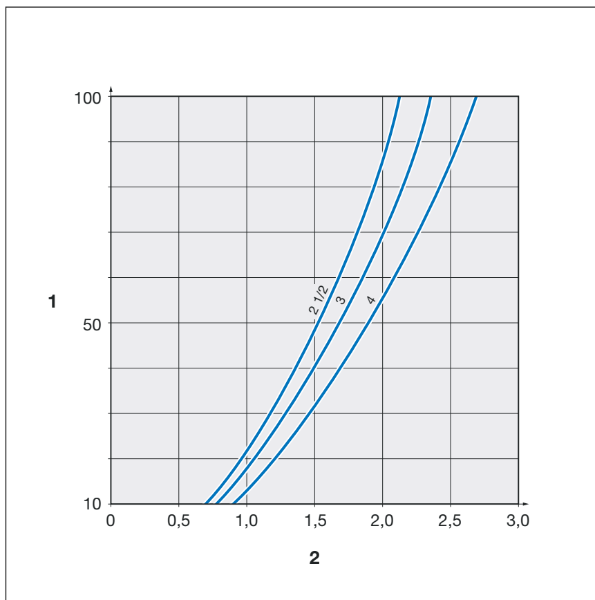
Afb. 7: Uitzettingsliër U-vorm voor Megapress S XL 2½ tot 4 duim
