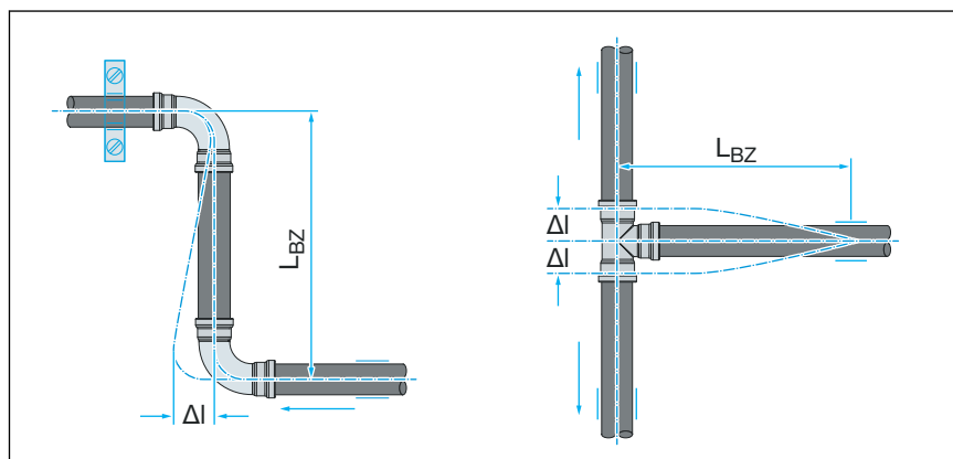
Afb. 4: Uitzettingsluis Z-vorm en T-vorm
