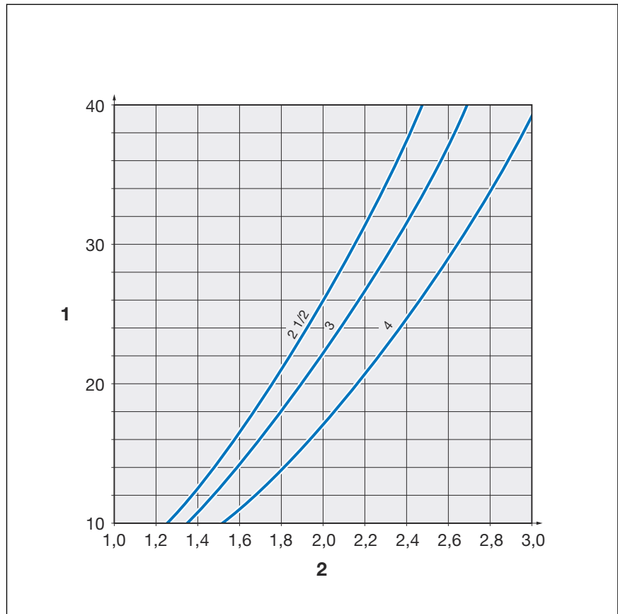
Afb. 5: Uitzettingslier Z-vorm en T-vorm voor Megapress S XL 2½ tot 4 duim
