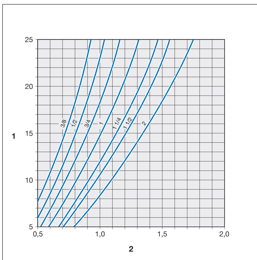
Afb. 5: Uitzettingsliër Z-vorm en T-vorm voor Megapress S 3/8 tot 2 duim
