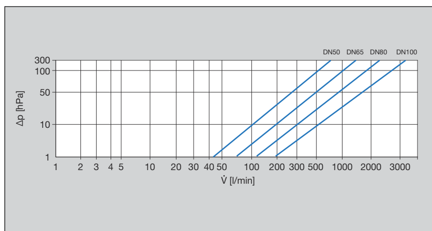
Afb. 1: Vermogensdiagram drukverlies KRV XL ventielen met schuine zitting flensaansluiting
