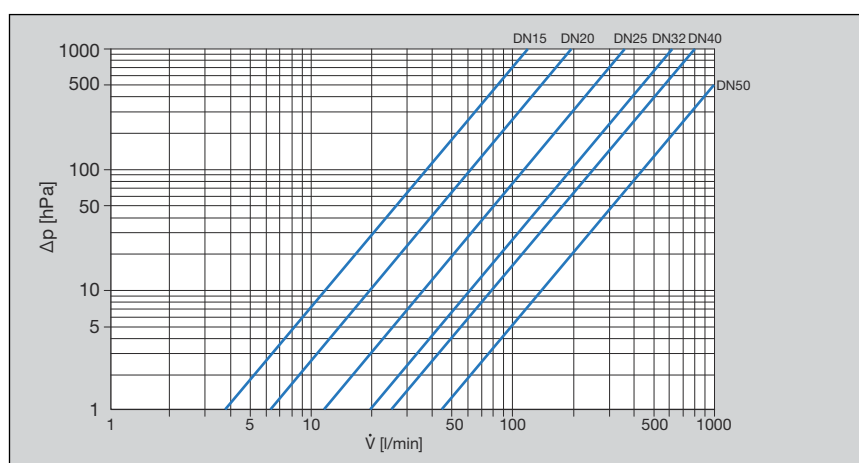
Afb. 1: Vermogensdiagram ventielen met schuine zitting pers-/draadaansluiting
