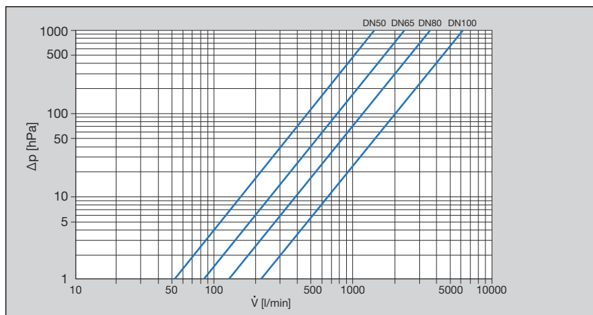
Afb. 1: Vermogensdiagram drukverlies XL ventielen met schuine zitting flensaansluiting
