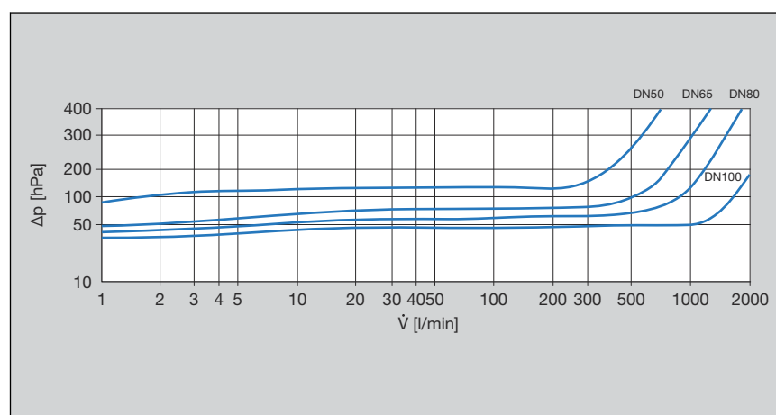
Afb. 1: Vermogensdiagram drukverlies terugstroomblokkeerklep flensaansluiting
