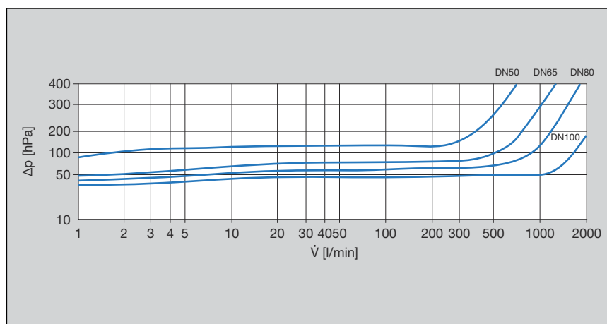
Afb. 1: Vermogensdiagram drukverlies terugstroomblokkeerlep flensaansluiting
