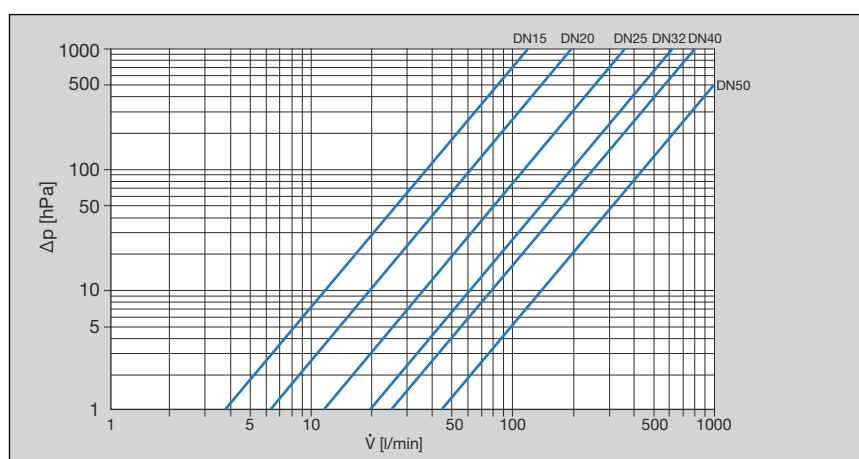
Afb. 1: Vermogensdiagram ventielen met schuine zitting pers-/draadaansluiting
