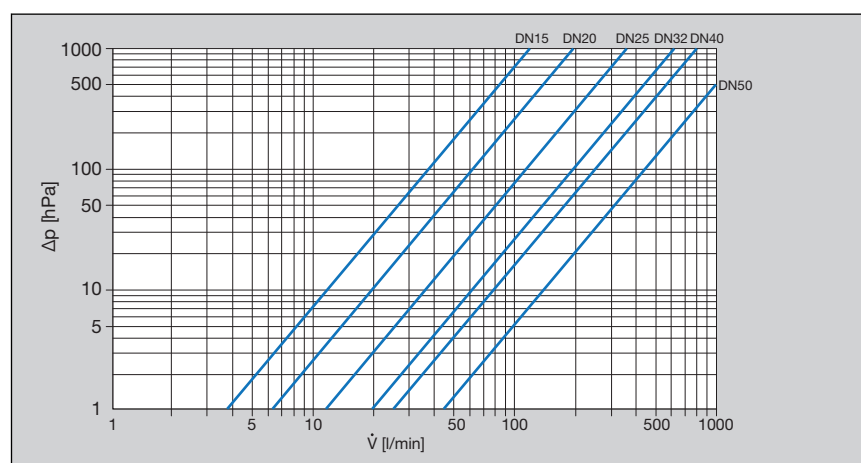
Fig. 2: Diagramma di prestazione valvole inclinate estremità a pressare femmina/filettata
