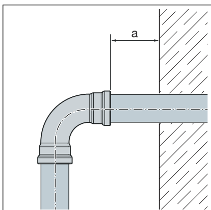
Minimális távolság D 2½–4 méretű présgyűrűk esetén
