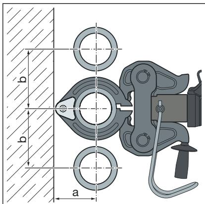
Helyigény, présgyűrűk D 2½–4
