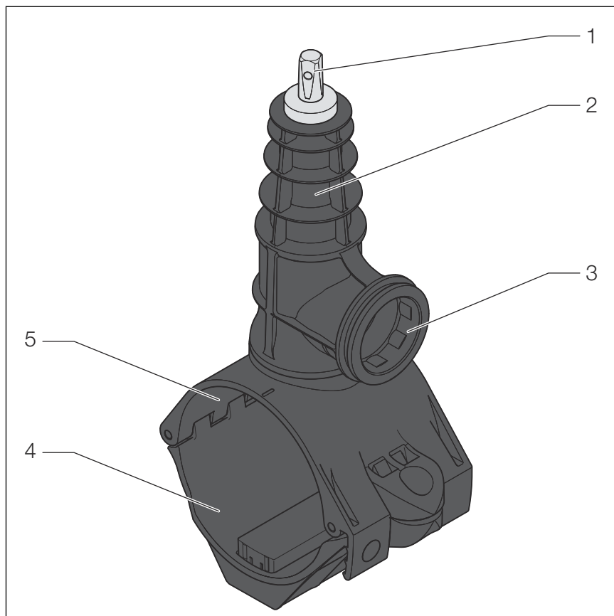
2. ábra: Megfúróidom alkatrészei
