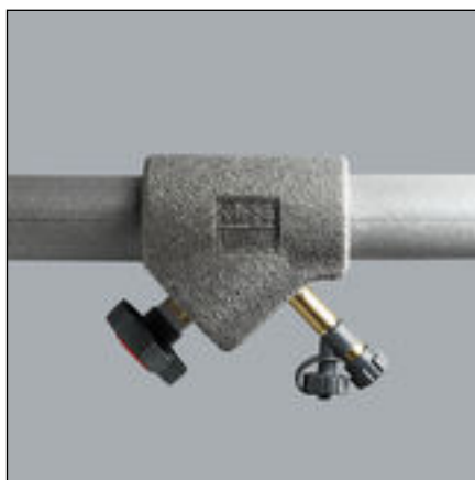
Slika 6: Easytop izolacijski kalup s produžetkom i ventilom za pražnjenje
