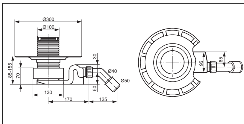
Fig. 6 : Schéma coté modèle 4927
