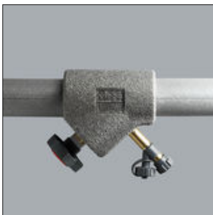
Fig. 6: Coque isolante Easytop avec prolongement et vanne de vidange
