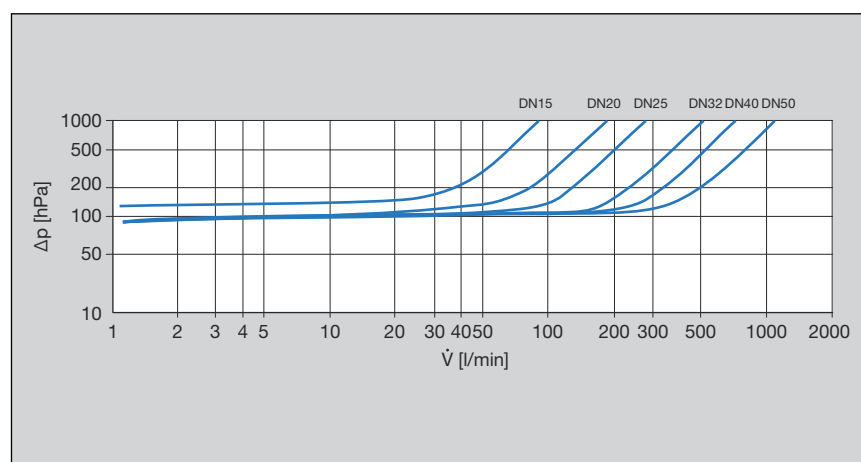
Fig. 3: Diagramme de performances perte de charge KRV raccord à sertir/raccordement fileté
