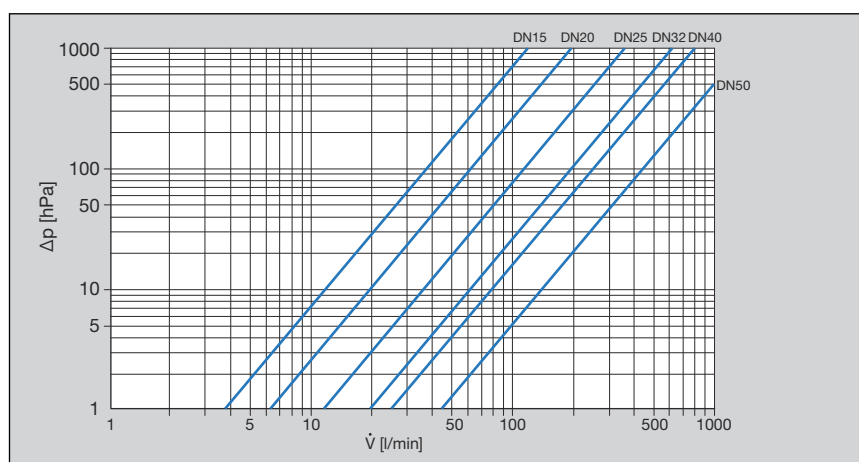
Fig. 3: Diagramme de performances vannes à siège incliné raccord à sertir/raccordement fileté
