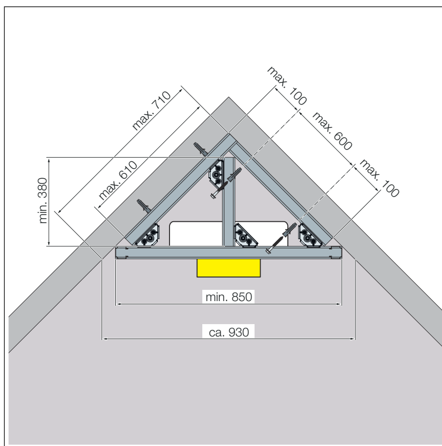
Fig. 8: Dimensions pour montage en angle
