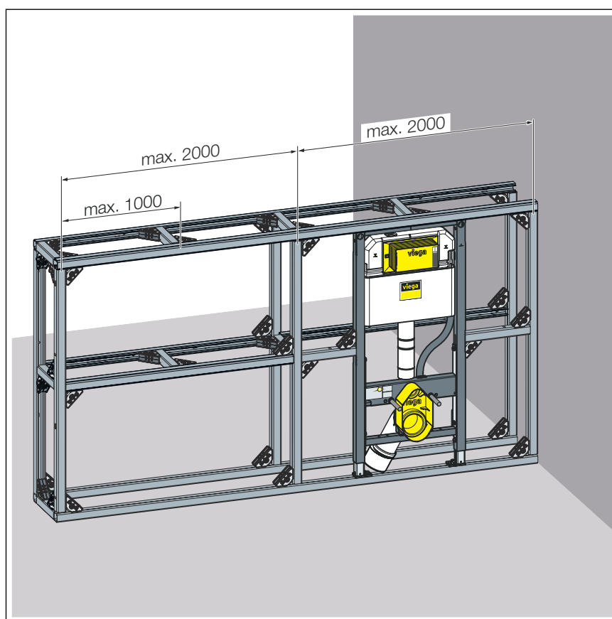
Fig. 10: Cotes de montage, séparation de pièce mi-haute avec élément (à raccord unilatéral)
