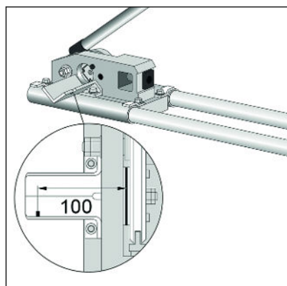
Fig. 23: Coupe-profilé Prevista Dry Plus
