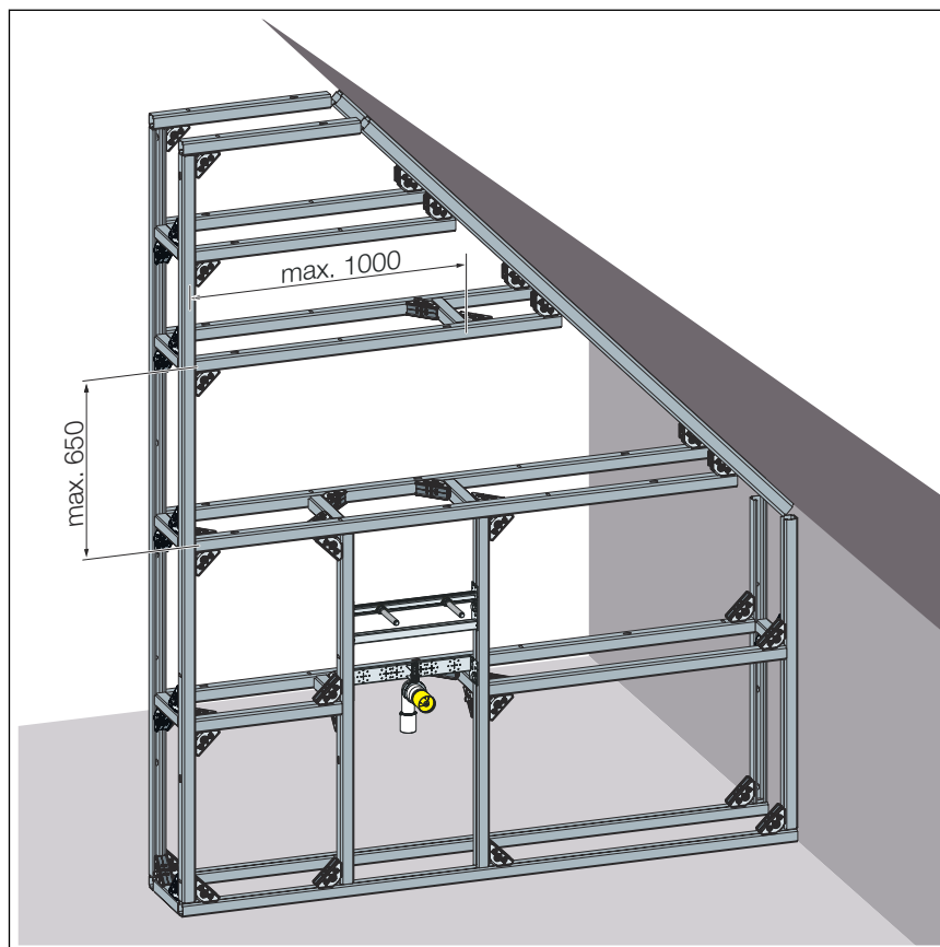
Fig. 16: Cotes de montage, cloison de séparation sur le pan du toit
