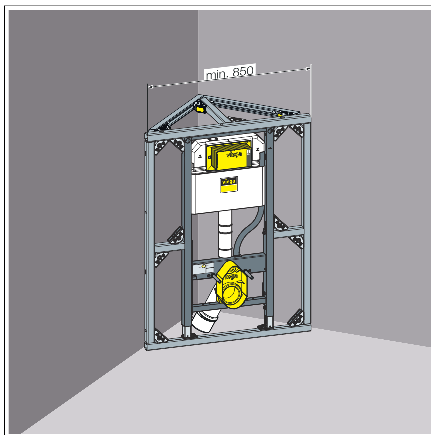
Fig. 7: Dimensions pour montage en angle
