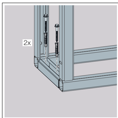
Fig. 20: Profilé de montage au sol
