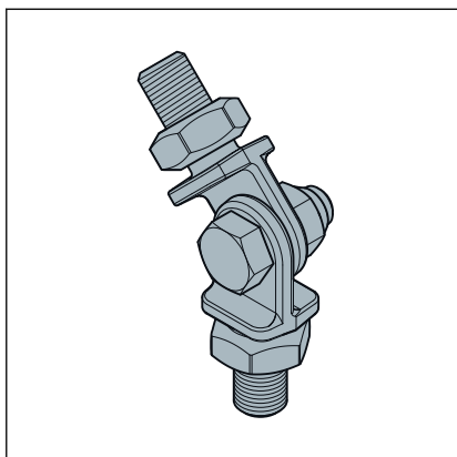
Fig. 17: Rotule de montage Prevista Dry Plus
