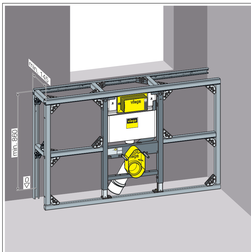
Fig. 12: Cotes de montage, hauteur de construction basse (actionnement par l'avant)
