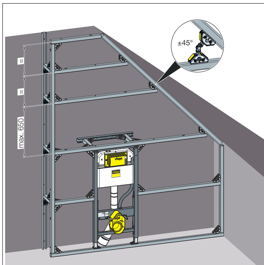
Fig. 15: Cotes de montage, bâti-support sur le pan du toit
