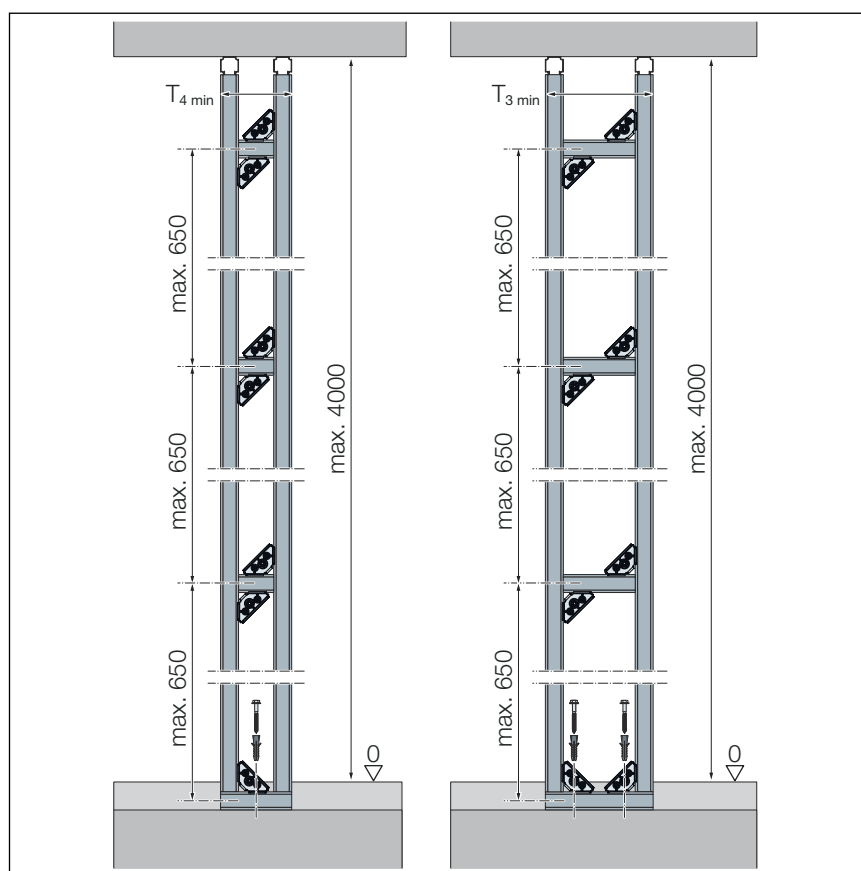
Fig. 25: Cloison de séparation
