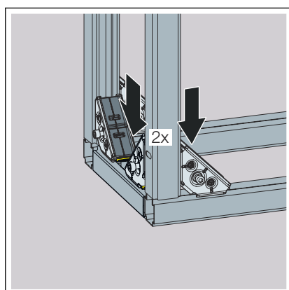
Fig. 21: Pièces de liaison en bas
