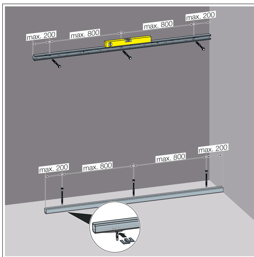
Fig. 31: Cotes fixation du profilé
