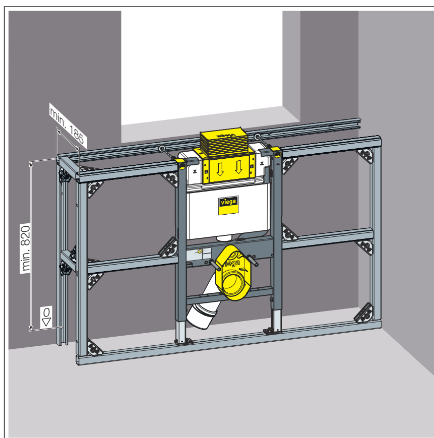
Fig. 13: Cotes de montage, hauteur de construction basse (actionnement par le haut)
