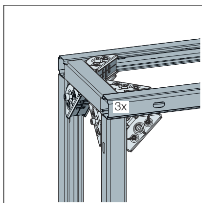
Fig. 22: Pièces de liaison en haut
