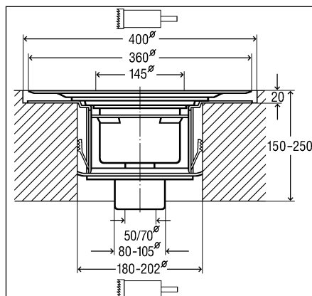
Fig. 7: Schéma coté pour modèle 4951.20
