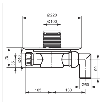
Fig. 7: Schéma coté pour modèle 4935.3
