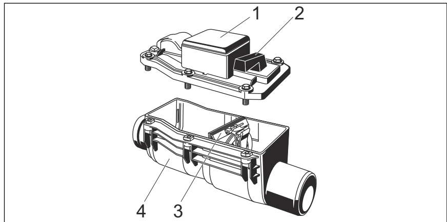
Fig. 3: Dispositif anti-retour Grundfix type 1
