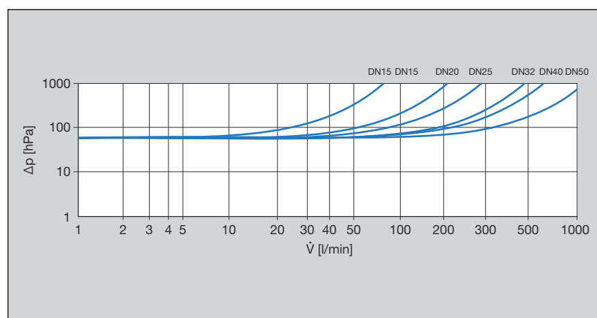
Fig. 1: Diagramme de performances perte de charge clapet anti-retour avec raccord à sertir/raccordement fileté
